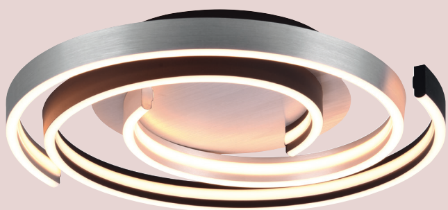
LED-DECKENLEUCHTE, Metall, Aluminium gebürstet, 1x 58W, 6800lm, 2300+3000+4000K, Ø ca. 50 cm, H: ca. 9 cm, dimmbar über Lichtschalter.
